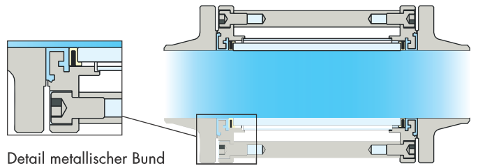
Detail metallischer Bund
